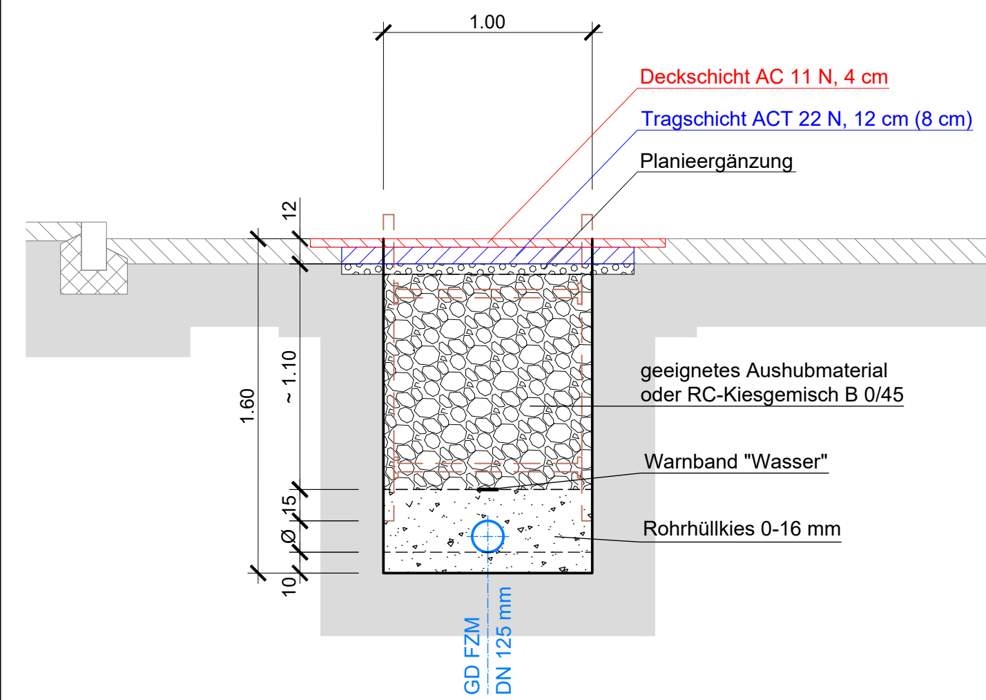
Grabenprofil 1:25
